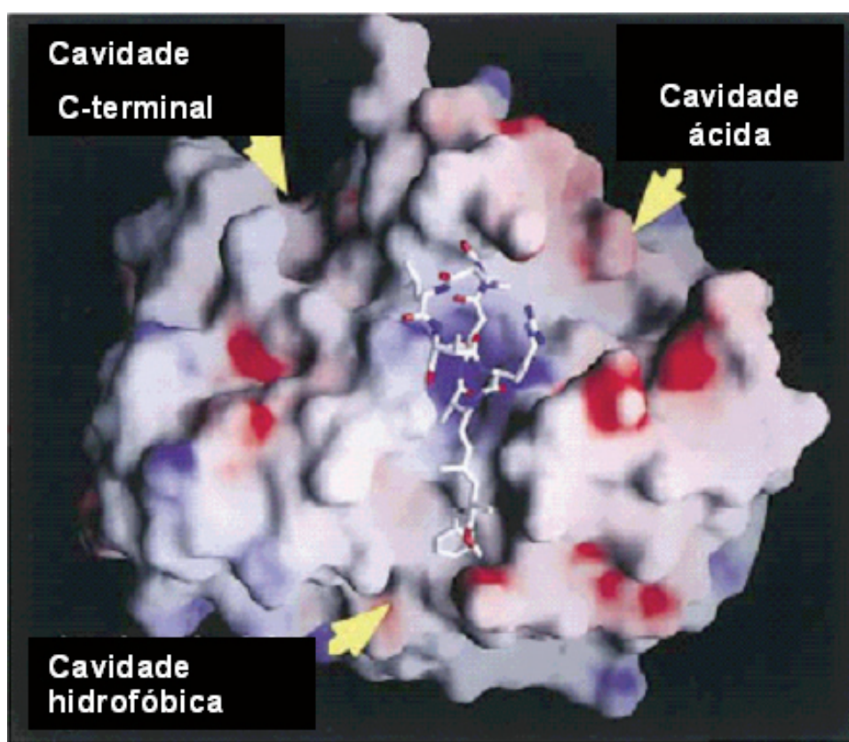
Figura 2. Superfície molecular do complexo PP1-MCYST-LR. No centro está a molécula de microcistina-LR com o aminoácido Adda ocupando o sítio ativo da enzima (na cavidade hidrofóbica). Fonte: Adaptado de Gupta et al. (1997).
